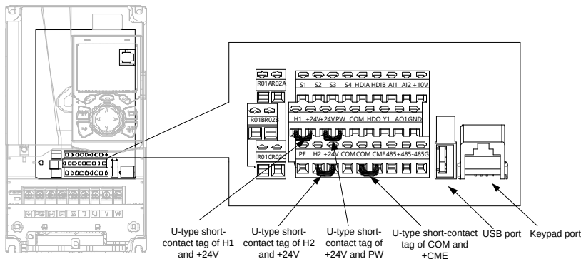
Рис 4.19 Расположение U-образных контактов
