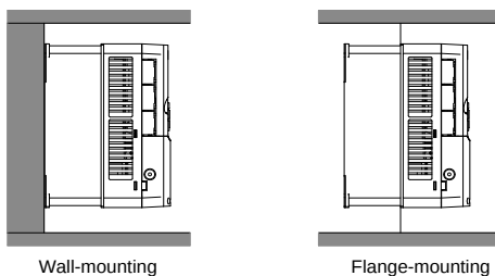
Рис 4.2 Способы установки
